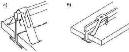
Рис. 49. Универсальная фиксирующая клипса BPA 7890 G (а), фиксирующая клипса BPA 819 G (б)
