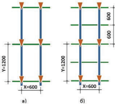
Рис. 16. Усиленная компоновочная схема: а) для плит 1200×600 мм и б) для плит 600×600 мм
