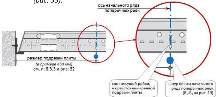
Рис. 33. Совмещение слота несущих реек с осью начального ряда поперечных реек
