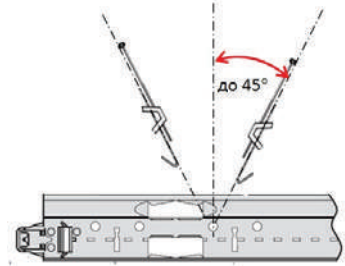
Рис. 36. Расположение подвесов вдоль оси несущей рейки
