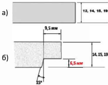
Рис. 4. Типы кромок плит а) Board, б) Tegular
