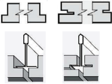
Рис. 6. Кромка Vector
