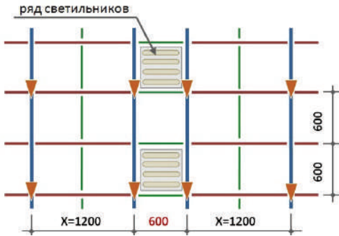
Рис. 17. Комбинированная компоновочная схема
